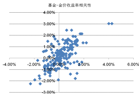
图 5：黄金相关共同基金与金价日收益率间相关性
